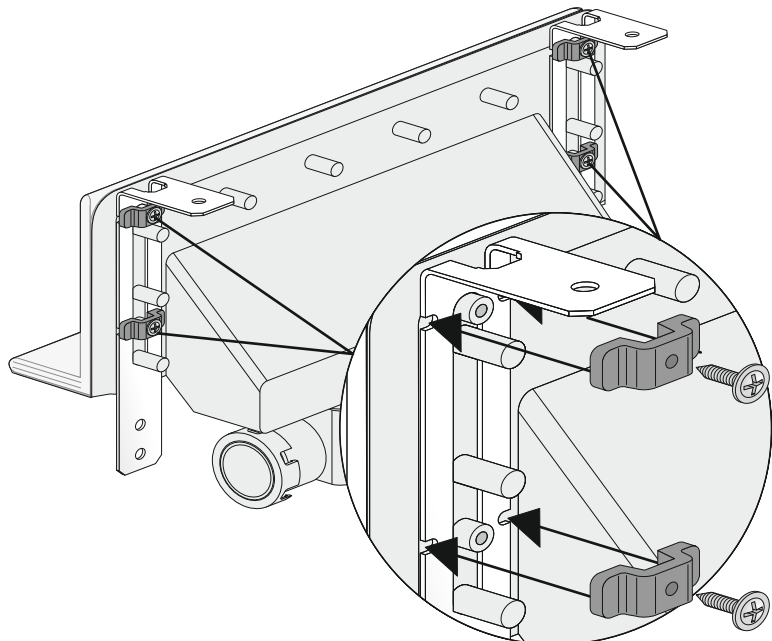
Unterputzwandbatterie 17.268.00.0000
