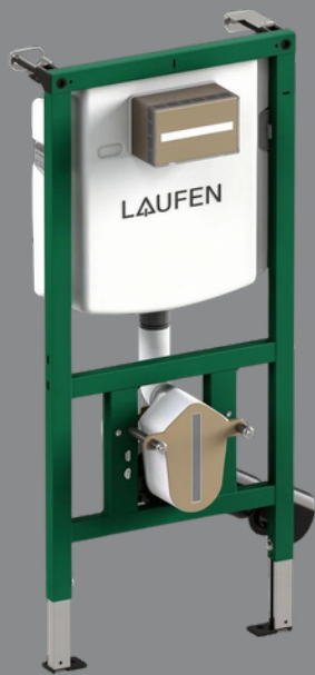
TOILET UNIT
