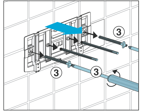
FRIAPLAN Art. 35 20 03
