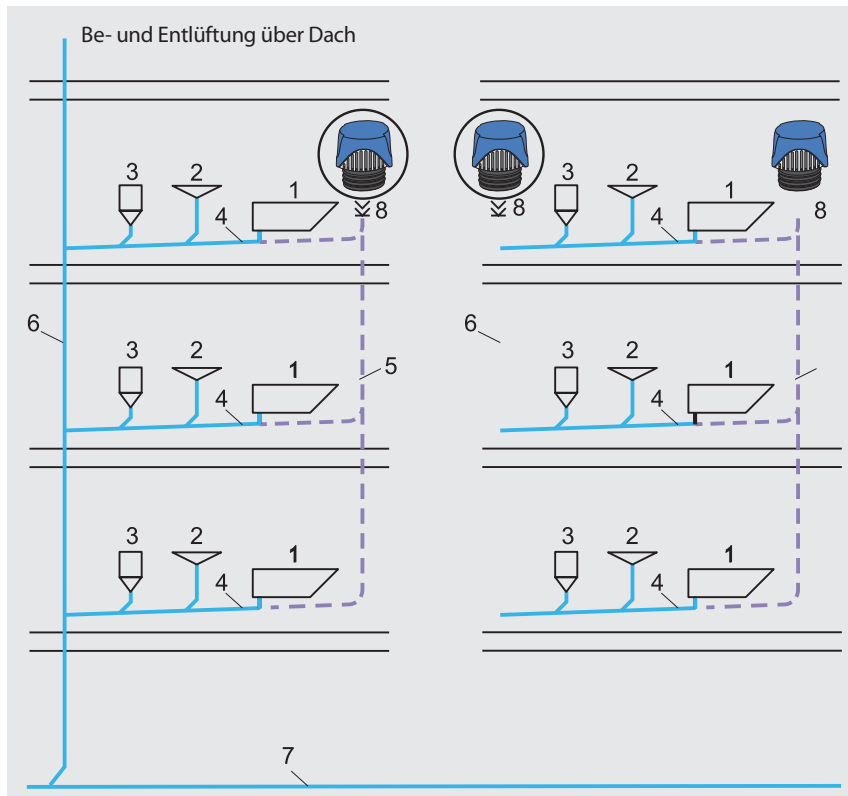
Belüftung von Fallleitungen mit ventilair®
