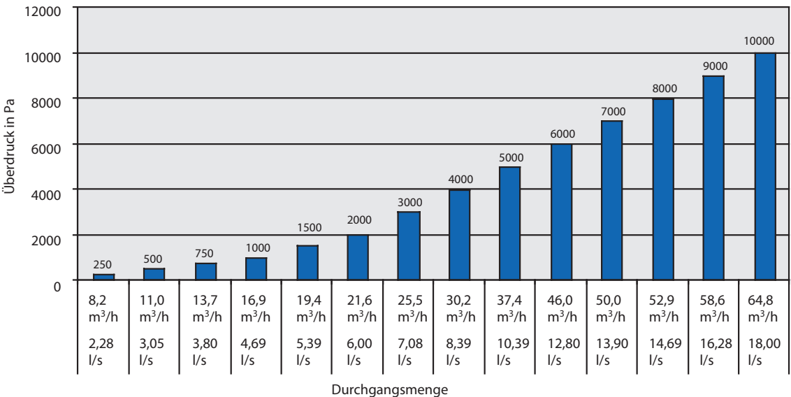
DIAGRAMM 1: Verhältnis Luftdurchgangsmenge – Überdruck, gemessen bei der TÜV Rheinland LGA Products GmbH
