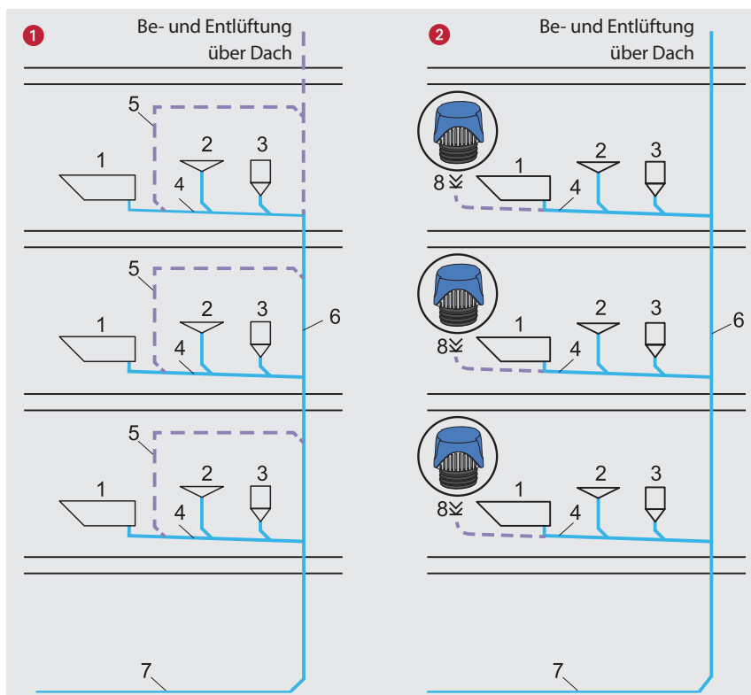
Belüftung von Sammelleitungen
