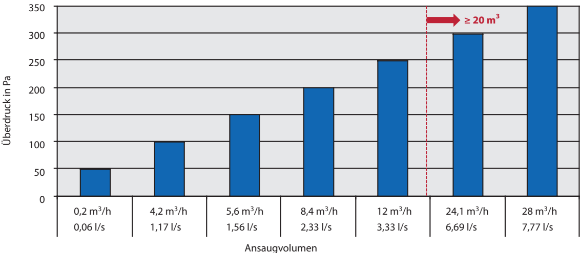
DIAGRAMM 2: Verhältnis Luftansaugvolumen – Unterdruck, gemessen bei der TÜV Rheinland LGA Products GmbH
